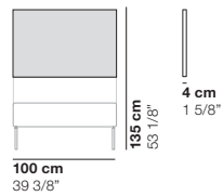
cod. 1212 / back panel 100 h. 135
