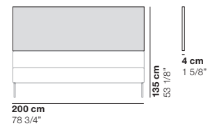
cod. 1216 / back panel 200 h. 135
