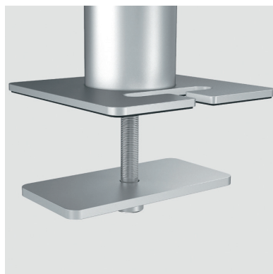
Bureaubevestiging met bladdoorvoer voor bureaudiktes van 14 tot 44 mm en bureaugatdiameters van 60 tot 80 mm.
