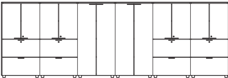
402,4 x 46 H.156,6 cm 158½" x 18" H.61¾" Armadio mod. ABA ABA Cabinet - Armoire ABA - Schränke ABA - Kasten ABA - Armario ABA
