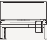
180 x 164 H.65÷130 cm 70¾" x 64½" H.25½"÷51" Composizione Bench Bench composition - Poste de travail - Bench-Arbeitsplatz - Samen- stelling bench - Composición bench
