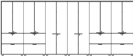
402,4 x 46 H.195 cm 158½" x 18" H.76¾" Armadio mod. ABA ABA Cabinet - Armoire ABA - Schränke ABA - Kasten ABA - Armario ABA
